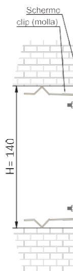
SEZIONE A-A
