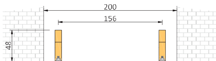
SEZIONE B-B
