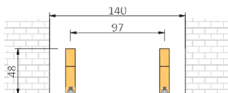
SEZIONE B-B
