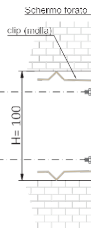
SEZIONE A-A
