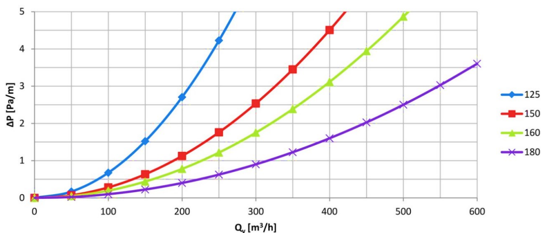
Grafické znázornenie tlakových strát
